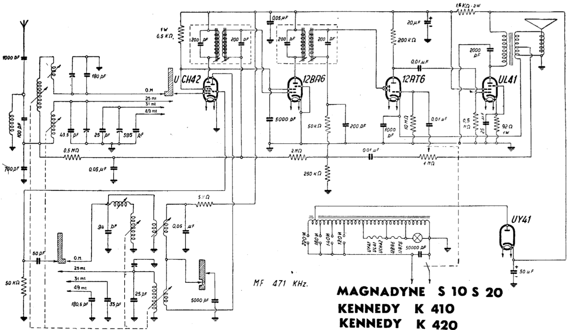
MAGNADYNE RADIO - Modd. MAGNADYNE S 10, S 20; KENNEDY K 410 e K 420. Una gamma onde medie e tre gamme onde corte. Sezione ad audiofrequenza con controreazione. Potenza di uscita 3 watt. Media frequenza 471 kc/s.
